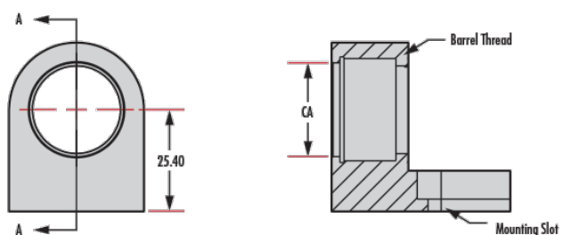
L-Slot Type (#36-410 & #36-416)
